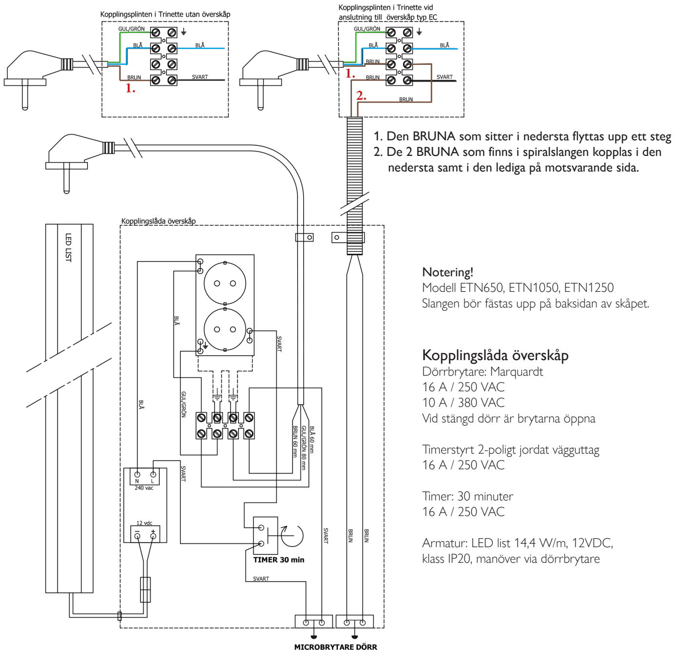
Kopplingsplint i Trinette utan överskåp
