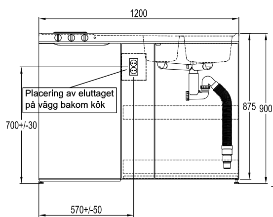
Minikök plåt 1200 mm
