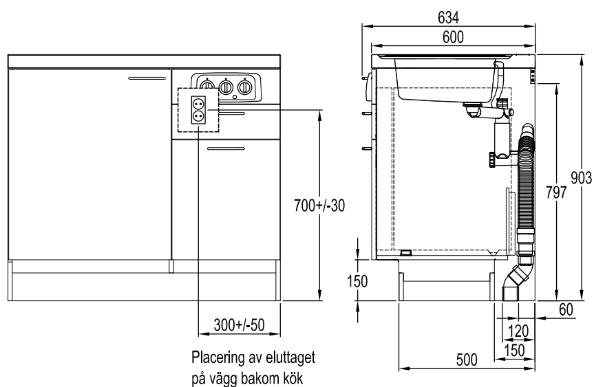
Trinette 1000 mm ETN1050, ETN1054, ETN1064
