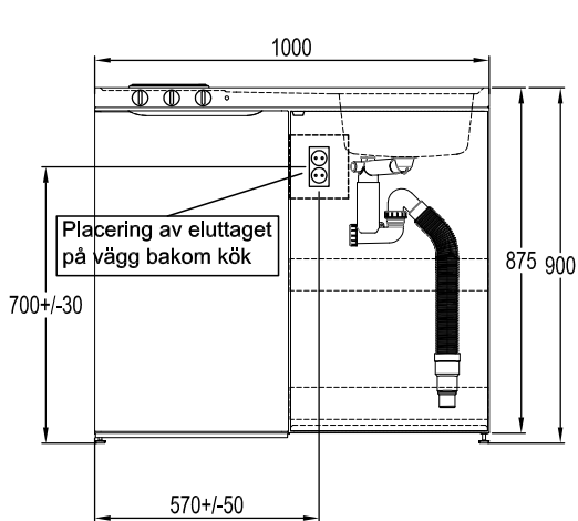
Minikök plåt 1000 mm
