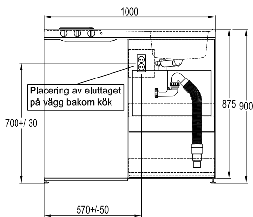
Minikök plåt 1000 mm
